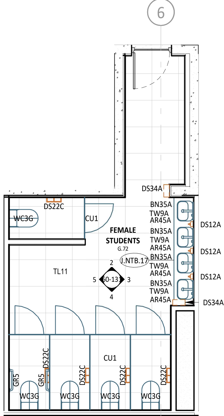
1 PLAN DETAIL 30-01 1 : 50
